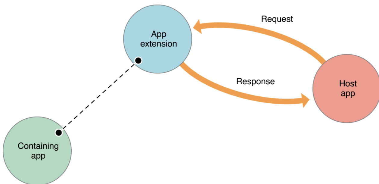
图 13-3 应用程序扩展、容器应用和宿主应用的通信
