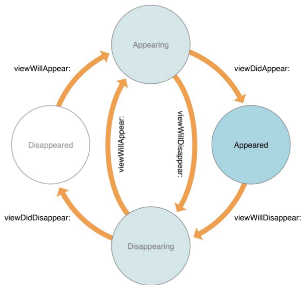
图 3-1 UINavigationController 不同状态的方法调用
