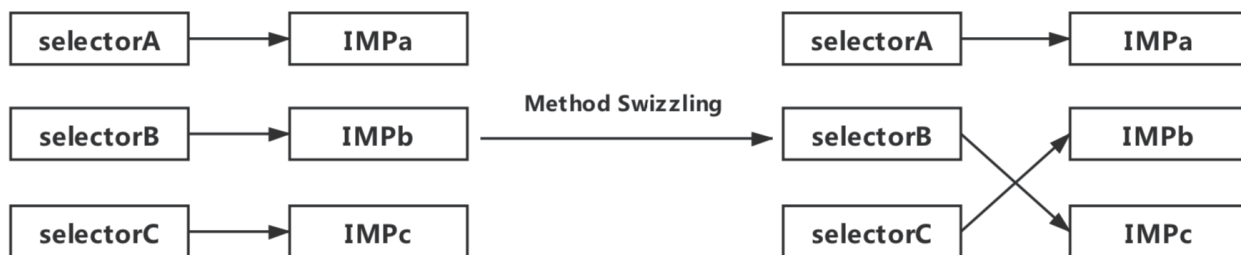
图 3-2 method_name 和 method_imp 映射关系
